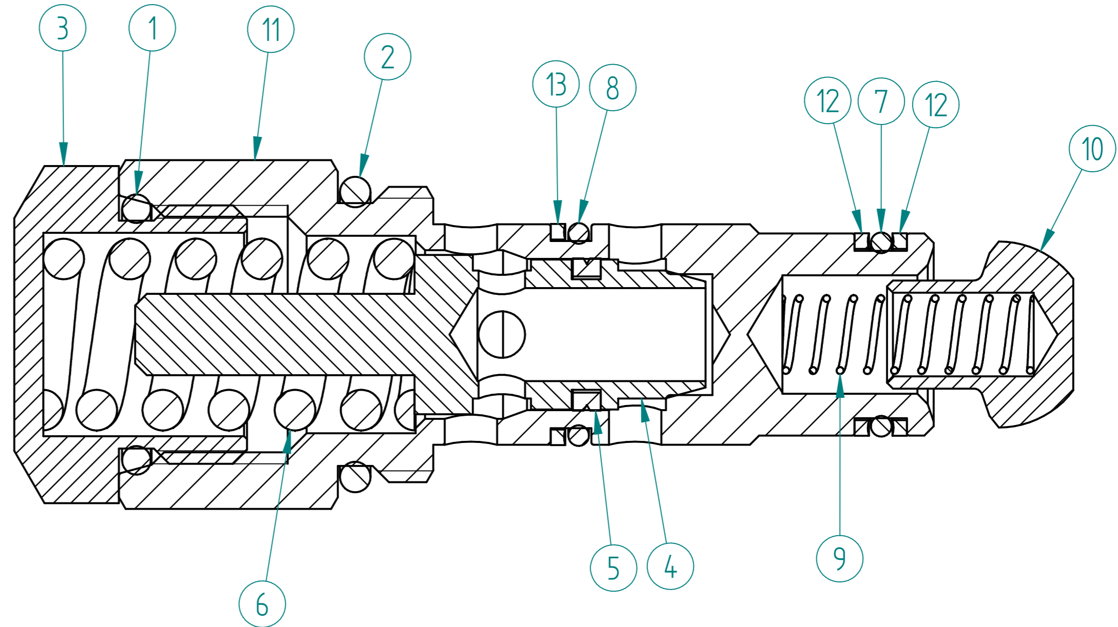
SECTION A-A
